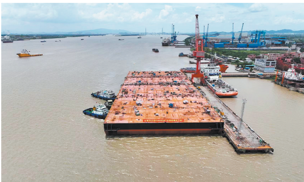
45000DWT半潜驳船主船体十分庞大,它的建造充分展现了我市“智”造实力。
