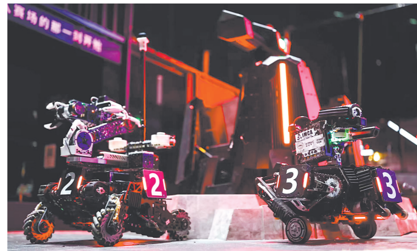
五邑大学IMCA战队研发的工程机器人(2号)和步兵机器人(3号)。活动主办方供图
